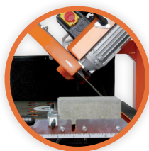
Coupe biseau 45°
