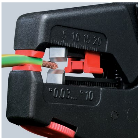
12 40 200: Dénudage précis sans endommagement du conducteur
