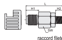
raccord fileté
