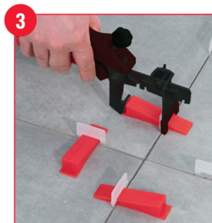
Serrage uniforme et constant grâce à la pince.
