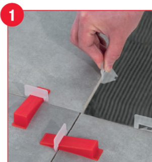
Mise en œuvre simple et rapide.
