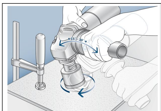
Puis continuer le perçage en décrivant un mouvement circulaire
