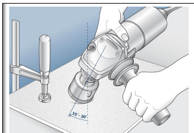
Amorce de perçage avec un angle de 15 à 30°
