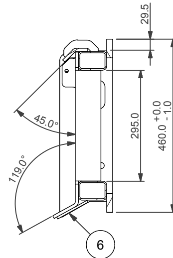
A-A (.1)
