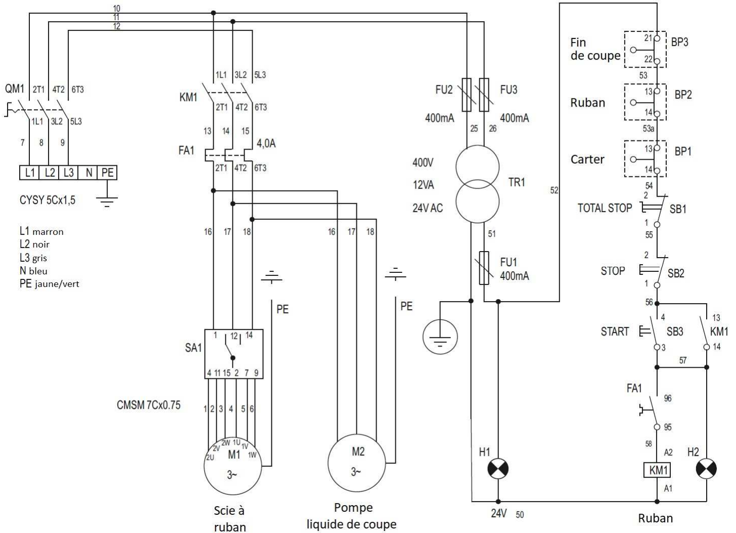
NOMENCLATURE SCHEMA ELECTRIQUE SR264DGDA (VUE 07)
