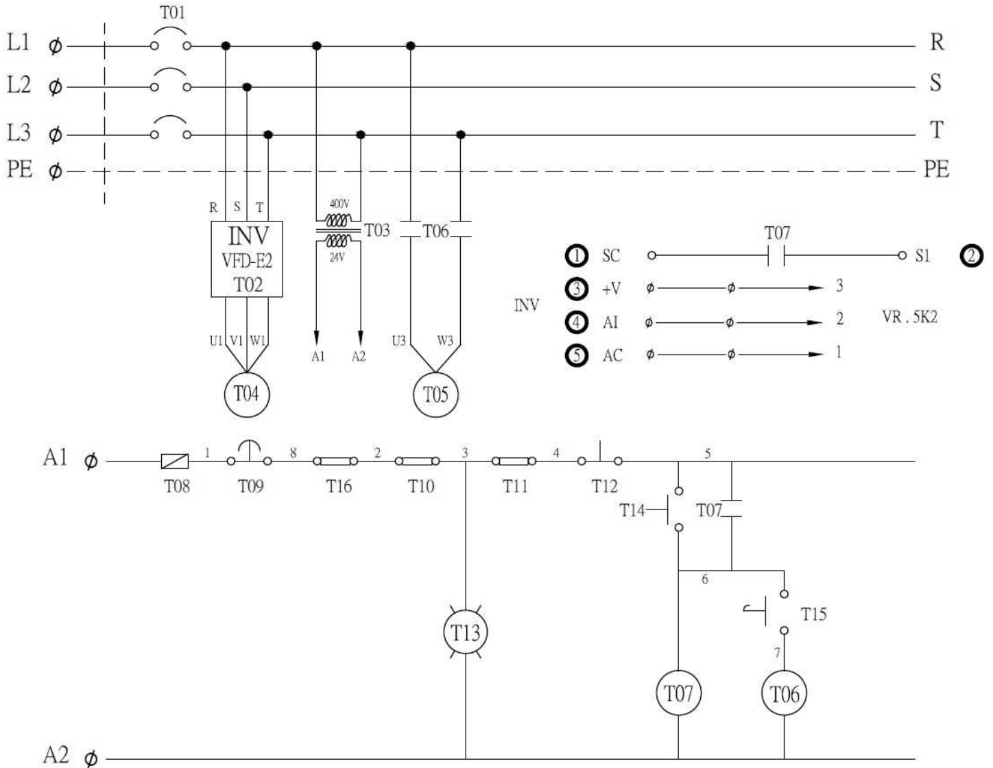
SCHEMA ELECTRIQUE SR276DGDAV (VUE 05)
