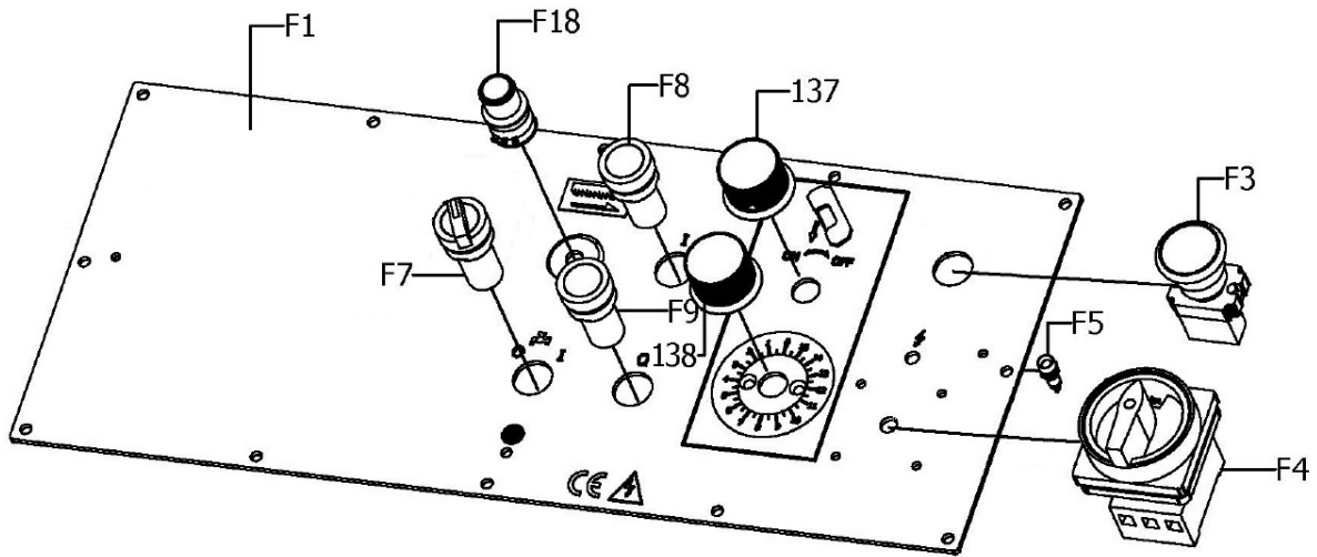
VUE ECLATEE ELECTRIQUE/HYDRAULIQUE SR276DGDAV (VUE 04)
