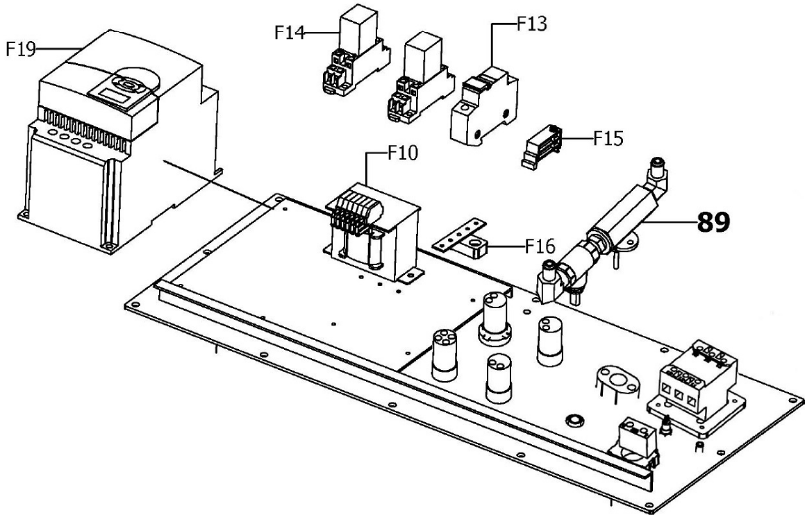
VUE ECLATEE ELECTRIQUE/HYDRAULIQUE SR276DGDAV (VUE 04)
