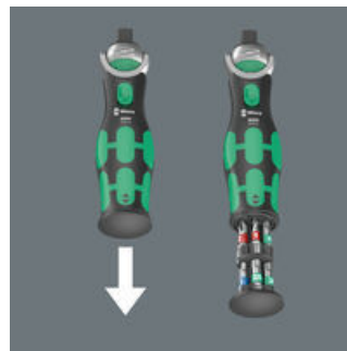
Le manche du cliquet compact Zyklop comprend une réserve captive pivotante pour 12 embouts (1/4", 25 mm de long).
